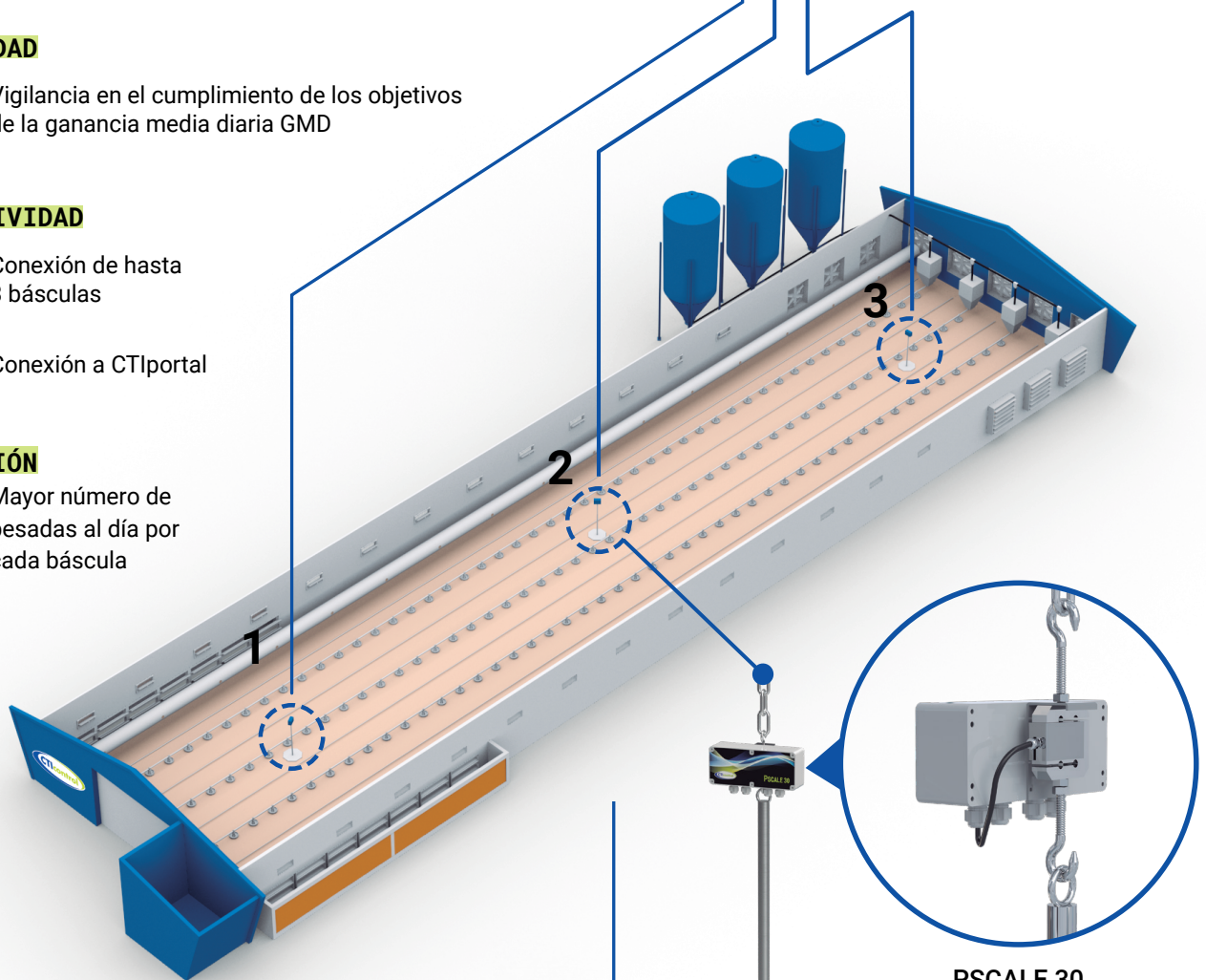
PLATAFORMA BÁSCULA
